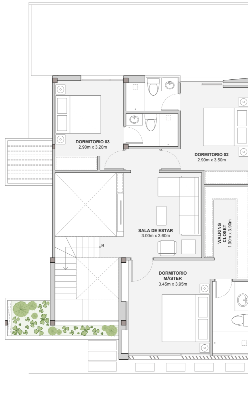
PLANTA ALTA
